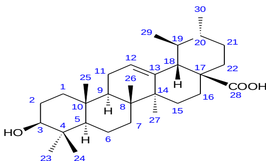
Şəkil 15. Ursol turşusunun ^1\text{H} və ^{13}\text{C} NMR spektroskopiya göstəricilərinə əsasən quruluşu
