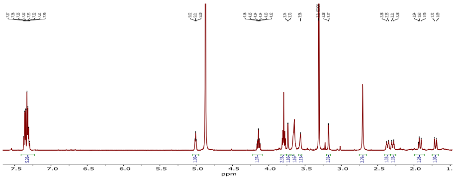
Şəkil 7. H. reticulatus -dan alınan skopolaminin ^1\text{H} NMR spektri
