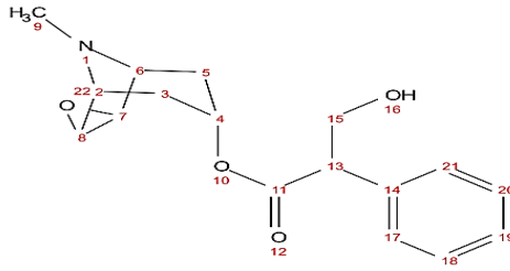
Şəkil 6. H. reticulatus -dan alınan skopolaminin ^1\text{H} və ^{13}\text{C} NMR spektrlərinə əsasən kimyəvi quruluşu
