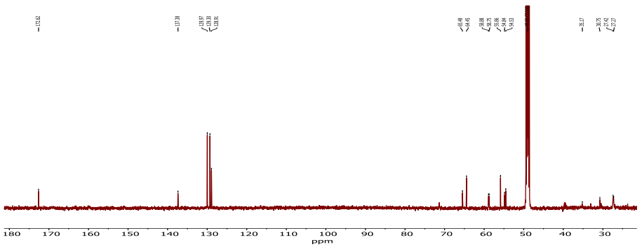
Şəkil 8. H. reticulatus -dan alınan skopolaminin ^{13}\text{C} NMR spektri
