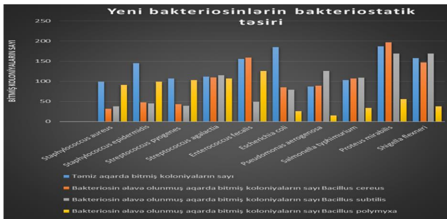
Şəkil 5.1. Bakteriosinlərin bəzi bakteriyaların bitməsinə bakteriostatik təsiri
