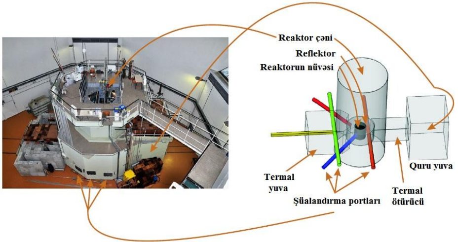
Şəkil 1. JSİ TRİGA Mark II reaktorunun üstdən fotosəkili və sxematik təsviri.
