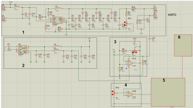
Şəkil 22. Qamma-spektrometrin elektron dövrəsi, 1-DC-DC gərginlik çevirici, 2-gərginlik invertoru(- gərginlik mənbəsi),3-siqnal gücləndirici, 4- komparator, 5-ARÇ MKA analizator və 6-personal kompyuter.
