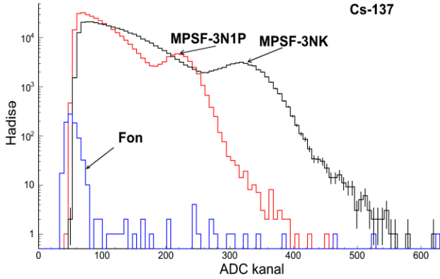
Şəkil 13. MSFD (3N1P və 3NK) fotodiod və plastik ssintilyator əsasında hazırlanmış detektorun ^{137}\text{Cs} izotopunun buraxdığı ionlaşdırıcı şüalanmanın amplitud spektri
