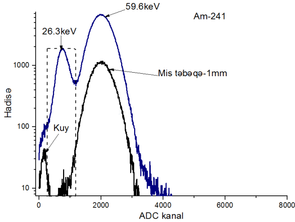
Şəkil 16. LFS-3 ssintilyator + MSFD fotodiod əsasında hazırlanmış detektorun 241 Am radioizotopundan qeyd etdiyi siqnalların amplitud paylanması.
