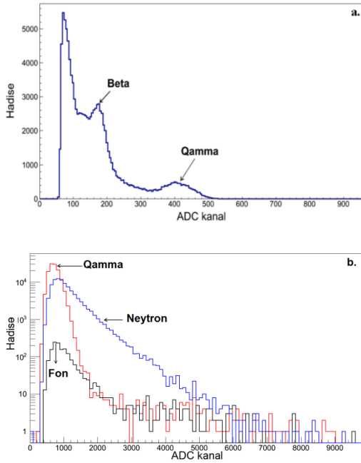
Şəkil 15. P-terfenil və stilben ssintilyatoru və MSFD-3N1P fotiodu ilə qeyd edilən beta zərrəciklərin, sürətli neytronların və qamma şüaların amplituda görə paylanma spektri.
