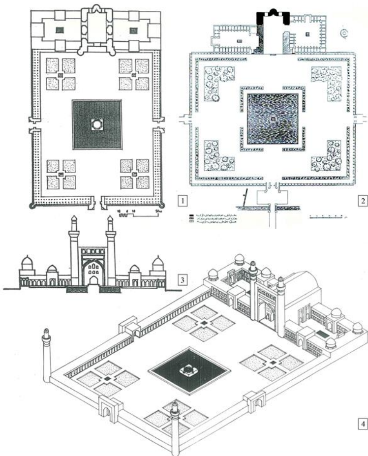
1,3,4- Əlişah məscidinin bərpə eskizi-plan, Ön və ümumi görünüşlər-(C.Qiası) 2- Əlişah məscidinin bərpə eskizi(D.Ulberdən)
