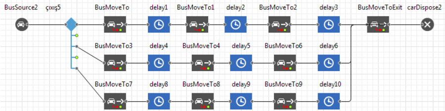
Şəkil 15. Eyni başlanğıc dayanacaqdan çıxan marşrutların simulyasiya alqoritmünün qurulması
