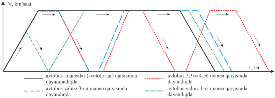
Şəkil 8. 4 svetofor obyektli marşrut sahəsində avtobusların hərəkət ssenariləri
