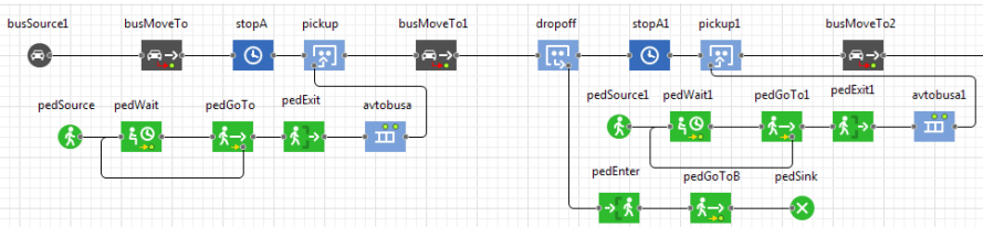
Şəkil 17. İki ardıcıl dayanacaqda sərnişinlərin minib-düşməsi modeli
