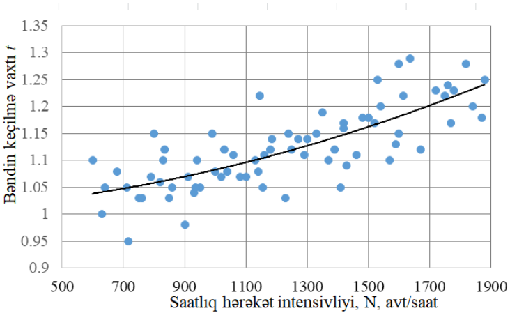
Şəkil 25. Real şəraitdə marşrut şəbəkəsinin bəndinin keçilmə vaxtının nəqliyyat axınının intensivliyindən asılı olaraq dəyişməsi
