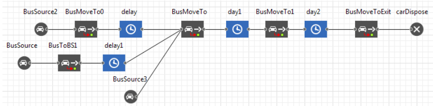
Şəkil 16. Dayanacaqları üst üstə düşən marşrutların simulyasiya alqoritminin qurulması
