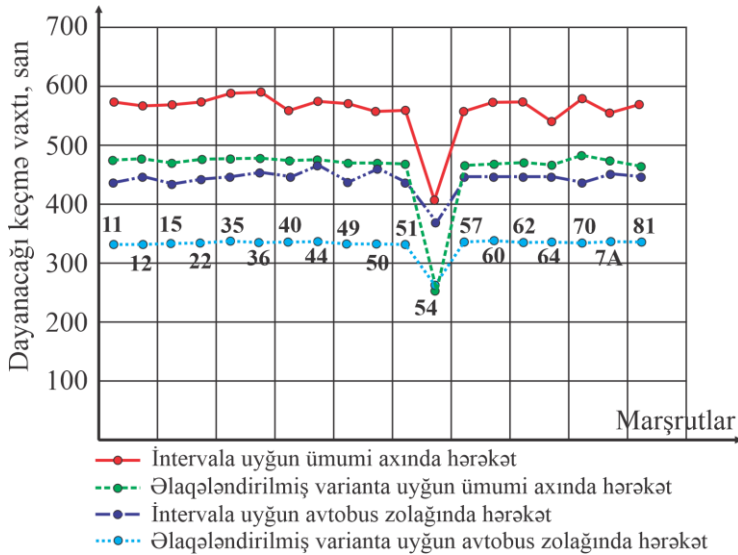
Şəkil 23. Ümumi axında və xüsüsüləşdirilmiş hərəkət zolağı üzrə avtobusların dayanacağı keçmə vaxtının paylanması
