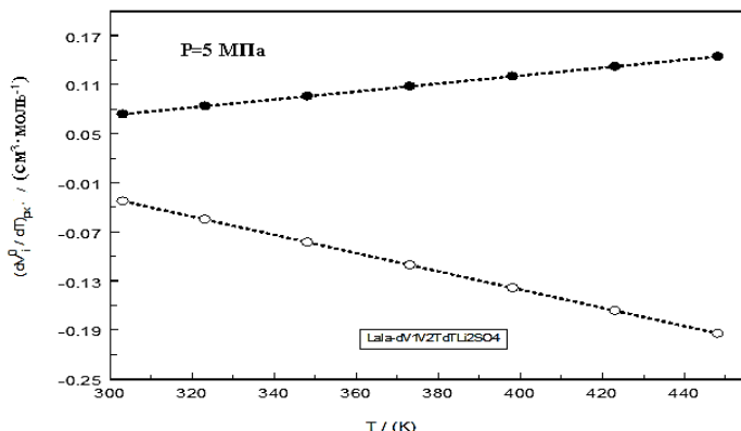
Рисунок 14. Рассчитанные значения коэффициента термического расширения парциальных молярных объемов \left(\partial \bar{V}_2^0 / \partial T\right)_{P\chi} соли \text{Li}_2\text{SO}_4 и \left(\partial \bar{V}_1^0 / \partial T\right)_{P\chi}
