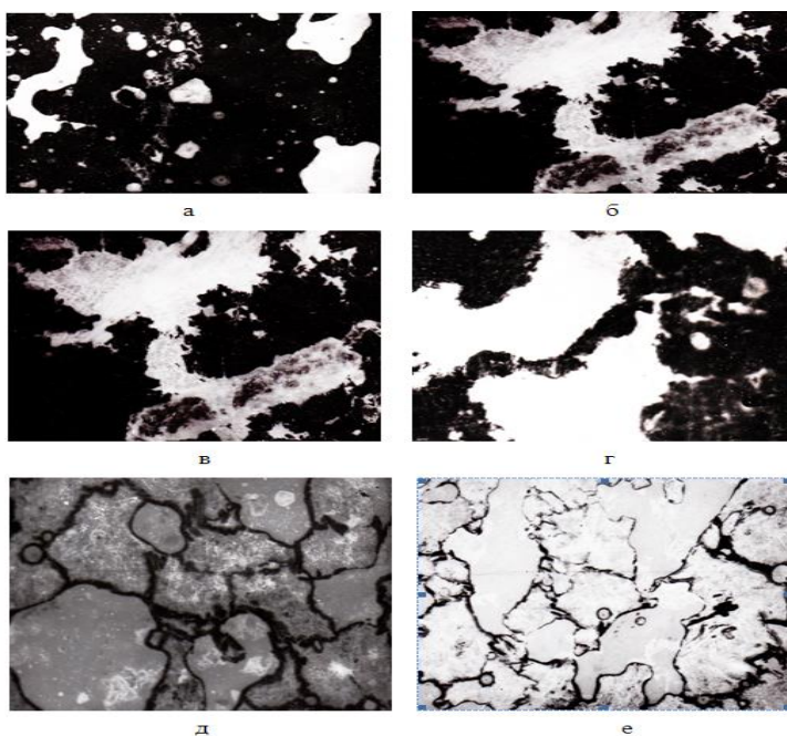
Рисунок 3. Микроструктура «железо-чугун-стекла», ×400: а, б; в, г; д, е; давление прессования 400;700 и 1000 МПа, соответственно, а, в, д; б, г, е содержание чугуна и стекла 10 и 2; 20 и 4 мас.%, соответственно
