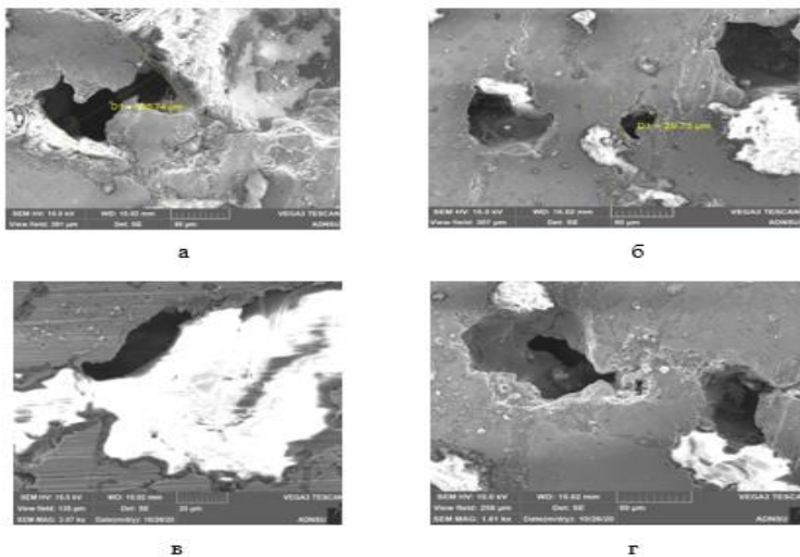
Рисунок 18. СЭМ-изображения распределения поры основной (а, в) и центральной (б, г) зон КМ «железо-чугун-стекло»
