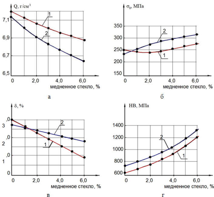
Рисунок 22. Зависимость плотности (а), предела прочности (б) относительного удлинения (в) и твердости (г) спеченных железо-чугун-стеклянных композиций: 1 – распыленный железный порошок; 2 – восстановленный железный порошок.
