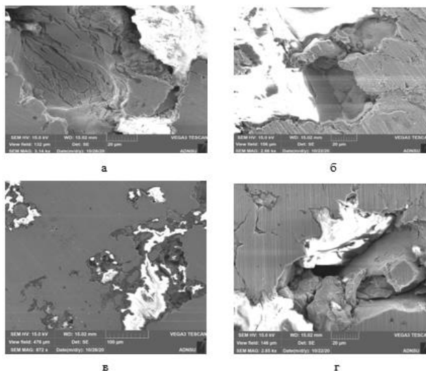
Рисунок 20. СЭМ- изображения траектории трещин по межкристаллитным границам чугуна-стекла (а, б) и участкам связующей фазы (железа) (в, г)
