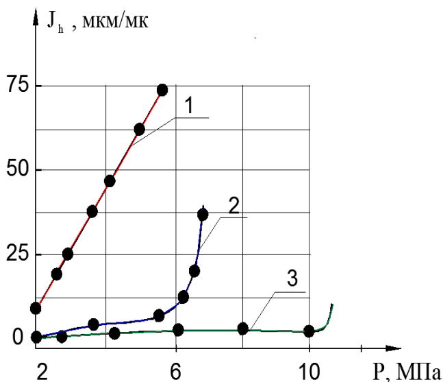
Рисунок 17. Зависимость интенсивности изнашивания от нагрузки трения порошковых бронз, содержащих медные порошки: 1 – 8 мас.% низкотемпературного стекла; 2 – 8 мас.% тугоплавкого оксида; 3 – по 6 мас.% стекла и оксида. V_{ск} = 1 м/с, трение без смазки пропитанных маслом образцов
