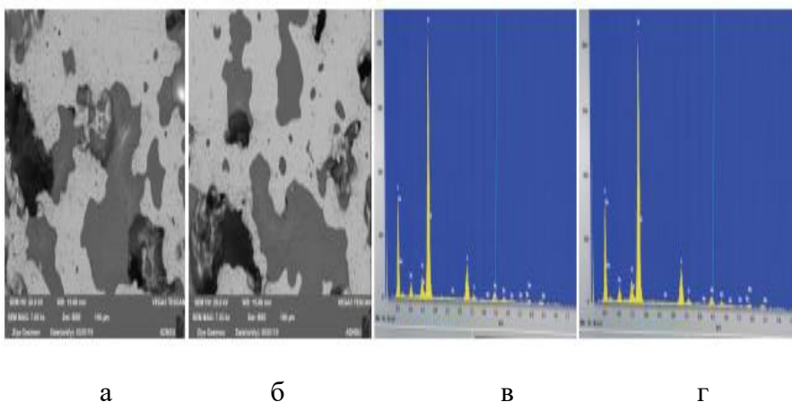
Рисунок 4. Насыщение частиц стекла Mn, Si и Fe-ом входивших в состав железо-, «железо-чугун-стеклянных» материалов:
