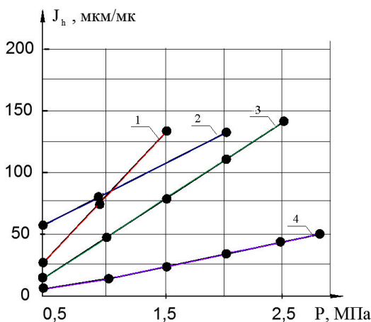
Рисунок 15. Зависимость интенсивности изнашивания от удельной нагрузки металлостеклянного материала различного состава (в массовых долях):
