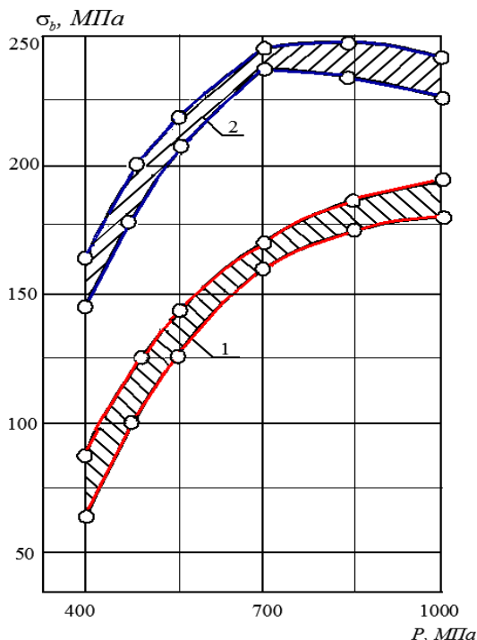
Рисунок 6. Зависимость \sigma_b от содержания чугуна и стекла в шихте и от давления прессования: 1; 2 – содержание чугуна и стекла в шихте 10; 20 и 2; 4 мас.% соответственно
