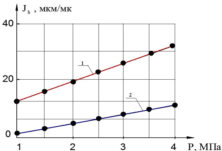
Рисунок 16. Зависимость интенсивности изнашивания от нагрузки трения порошковых материалов: 1 – бронза с 6 мас.% стекла и 30 мас.% чугуна (оба порошка не металлизированы); 2 – бронза с 6 мас.% стекла и 30 мас.% чугуна (оба порошка медненные); V_{ск} = 1 м/с, трение без смазки пропитанных маслом образцов.
