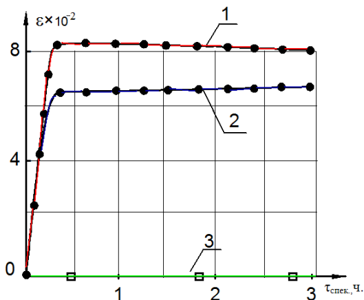
Рисунок 28. Зависимость относительной усадки железостеклянных прессовок от исходного размера порошка медненного чугуна: r = 50 \text{ мкм} (1), 100 \text{ мкм} (2) и 160 \text{ мкм} (3)
