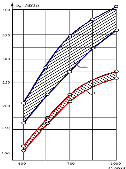
Рисунок 7. Зависимость \sigma_n материалов от содержания чугуна и стекла в шихте и давления прессования: 1; 2 – содержание чугуна и стекла в шихте 10; 20 и 2; 4 мас.% соответственно
