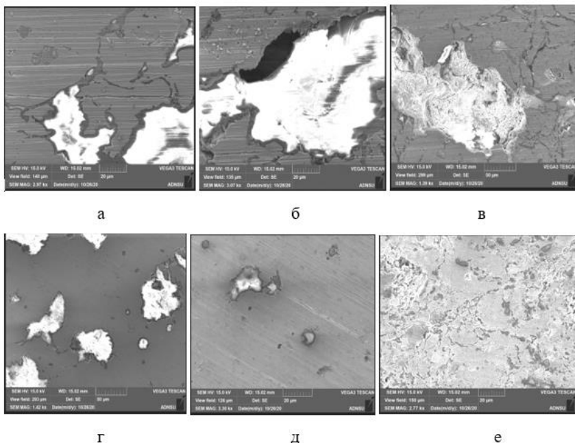
Рисунок 5. Изменение формы стеклянных частиц в процессе спекания: а, б; в, г; д, е; давление прессования 400;700 и 1000 МПа, соответственно, а, в, д; б, г, е содержание чугуна и стекла 10 и 2; 20 и 4 мас.%, соответственно.
