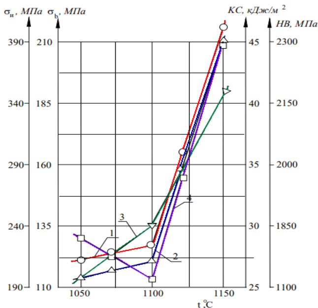
Рисунок 10. Зависимость механических свойств материала ЖЧ50С6 от температуры спекания: 1 - \sigma_b ; 2 - \sigma_n ; 3 – КС; 4 – НВ.
