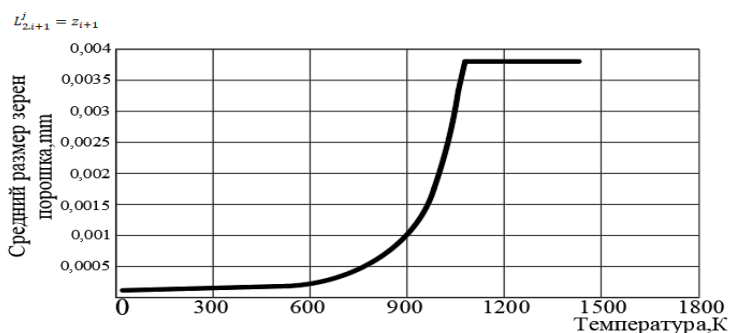
Рисунок 14. Зависимость среднего размера зерен порошка от температуры
