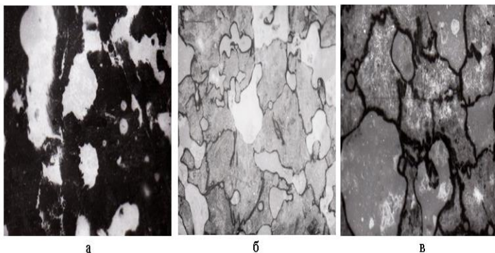
Рисунок 25. Микроструктура композиционного материала «железо-чугун-стекло», (20%.мас. медненный чугун, 4%.мас. медненное стекло и остальное железо ), \times 500 : а– P=400 МПа, t_{\text{спек.}}=1150 °С, \tau_{\text{спек.}}=1 ч.; б– P=700 МПа t_{\text{спек.}}=1150 °С, \tau_{\text{спек.}}=1 ч.; в– 1000 МПа, t_{\text{спек.}}=1150 °С, \tau_{\text{спек.}}=1 ч.
