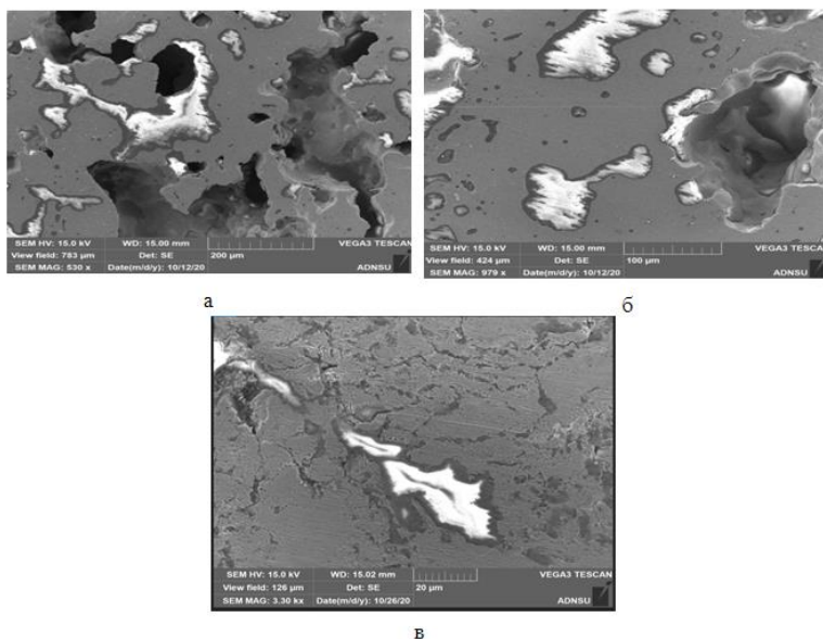
Рисунок 11. Образование в структуре крупных скоплений стекла при продолжительности спекания 3 часа: а-ЖЧ10С2; б-ЖЧ20С4; в-ЖЧ50С6
