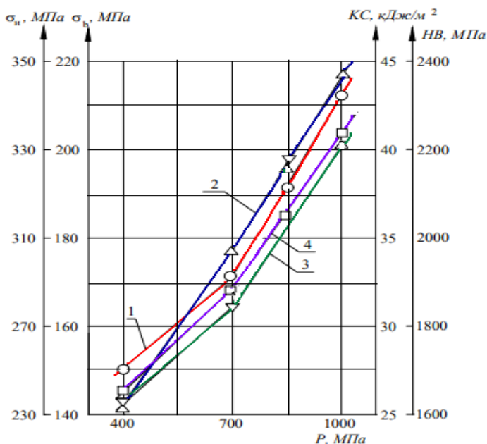
Рисунок 9. Зависимость механических свойств материала ЖЧ50С6 от давления прессования: 1 - \sigma_b ; 2- \sigma_n ; 3 – КС; 4 – НВ
