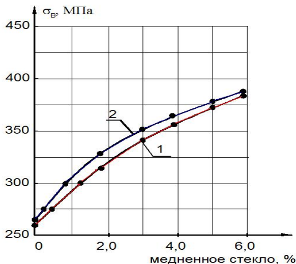
Рисунок 23. Зависимость прочности железо чугунастеклянных композиций после закалки и низкотемпературного отпуска: 1,2 – закалка, 900°С, вода; 1 – распыленный порошок; 2 – восстановленный порошок.
