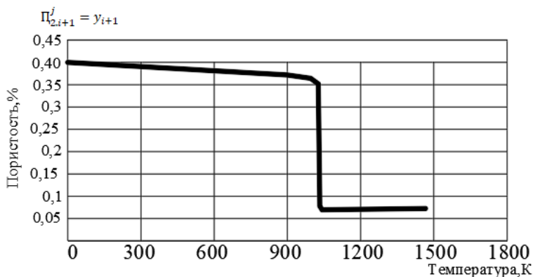
Рисунок 13. Зависимость пористости от температуры
