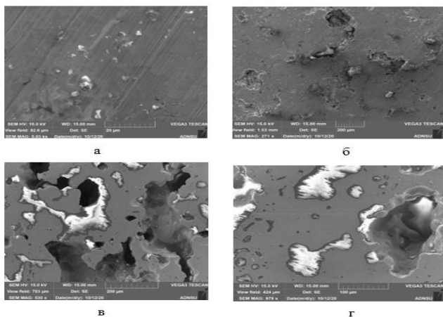
Рисунок 19. СЭМ-изображения распределения в структуре матрицы твердых включений меденного чугуна (а, б) и меденных включений стекла (в, г) в КМ «железо-чугун-стекло»
