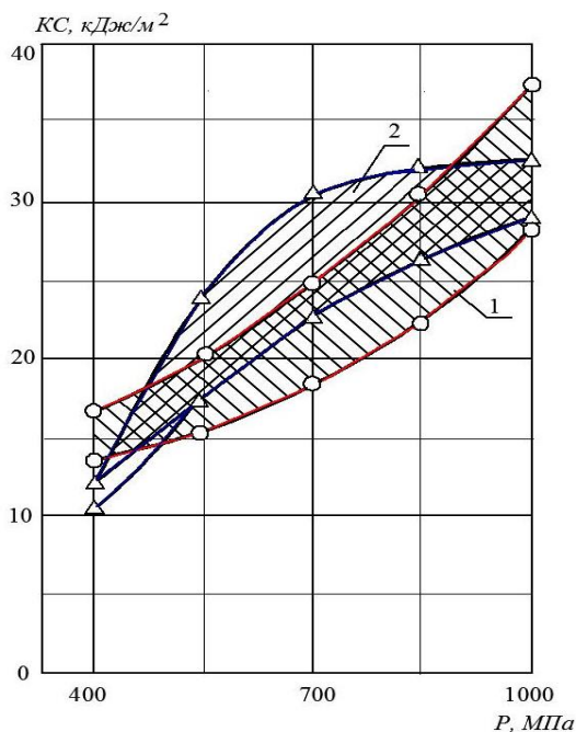
Рисунок 8. Зависимость КС материалов от содержания чугуна и стекла в шихте и давления прессования: 1; 2 – содержание чугуна и стекла в шихте 10; 20 и 2; 4 мас.% соответственно
