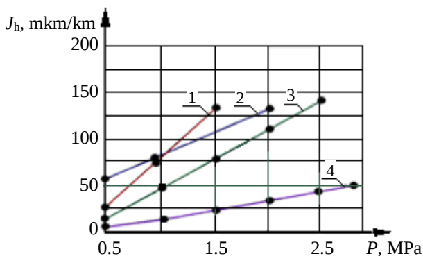
Şəkil 15. Müxtəlif tərkibdə (kütə, % nisbətində) metalşüşə materialının yeyilmə intensivliyinin mütləq yüklənmədən asılılığı:
