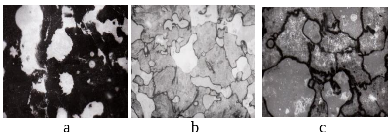
Şəkil 25. Dəmir-çuqun-şüşə kompozisiya materialının mikrostrukturu (20 küt.% mislənmiş çuqun, 4çək.% mislənmiş şüşə və qalanı dəmir x500):
