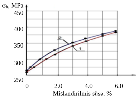
Şəkil 23. Dəmir-çuqun-şüşə kompozitinin tablandırımdan və aşağı temperaturlu tabəksiltmədən sonra möhkəmliyinin mislənmiş şüşənin miqdarından asılılığı:
