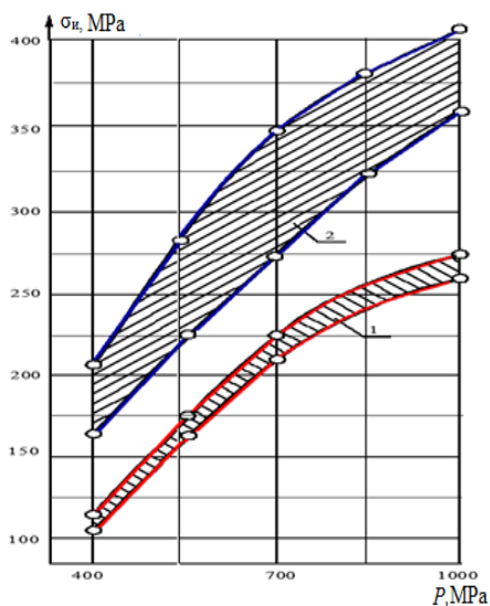
Şəkil 7. Materialların \sigma_u nin şıxtədə çuqun və şüşənin miqdarından və presləmə təzyiqindən asılılığı: 1; 2 – şıxtədə uyğun olaraq çuqunun və şüşənin miqdarı 10; 20 və 2;4 küt.%
