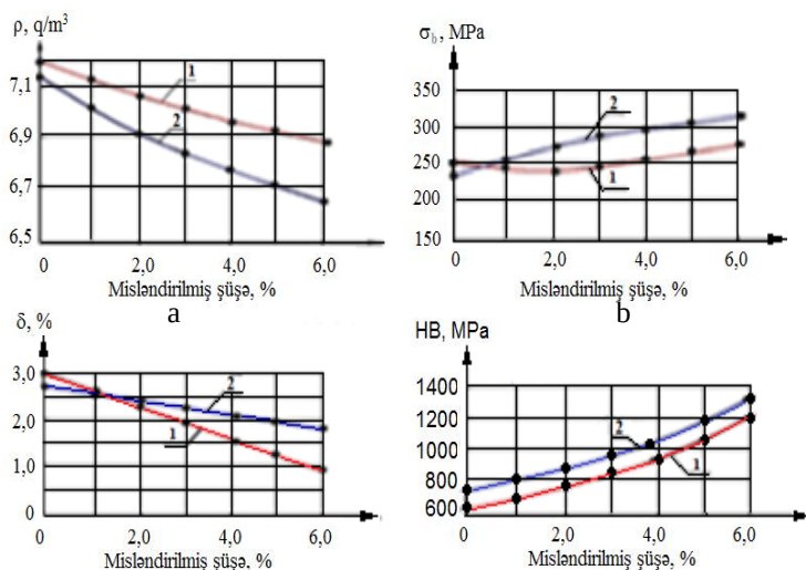
Şəkil 22. Bıxırılmış dəmir-çuqun-şüşə kompozisiyanın sıxlığının (a), möhkəmlik həddinin (b), nisbi uzanmasının (c) və bərkliyinin (d) mislənmiş şüşə ovuntusunun miqdarından asılılığı:
