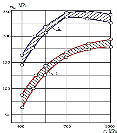
Şəkil 6. Materialların \sigma_b nin şıxtədə çuqun və şüşənin miqdarından və presləmə təzyiqindən asılılığı: 1, 2 – şıxtədə uyğun olaraq çuqunun və şüşənin miqdarı 10;20 və 2;4 küt.%
