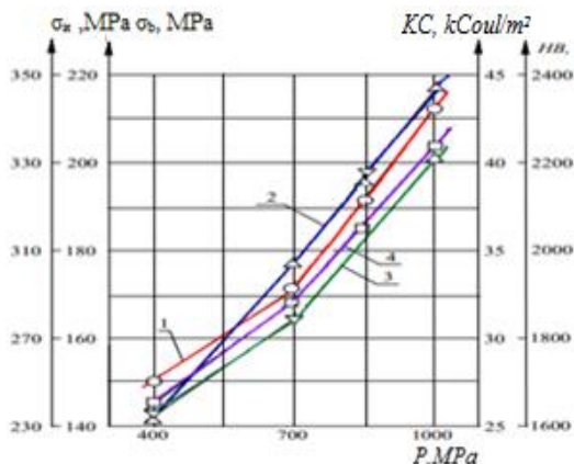
Şəkil 9. ЖЧ50С6 materialının mexaniki xassələrinin presləmə təzyiqindən asılılığı:
