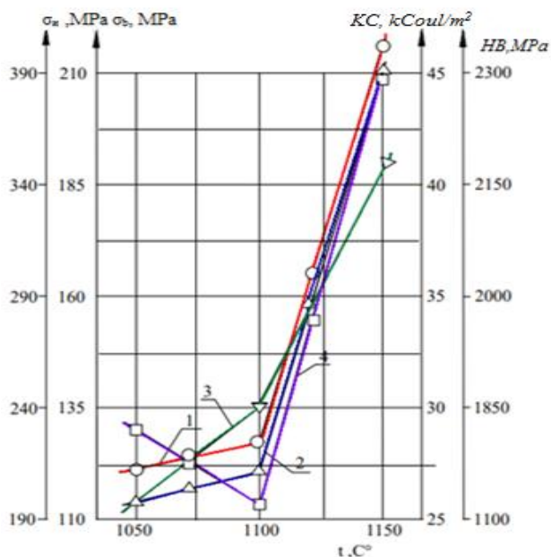
Şəkil 10. JC450C6 materialının mexaniki xassələrinin bişirmə temperaturundan asılılığı:
