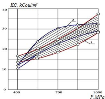
Şəkil 8. Materialın “KC”-nin şıxtədə çuqunun və şüşənin miqdarından və presləmə təzyiqindən asılılığı:
