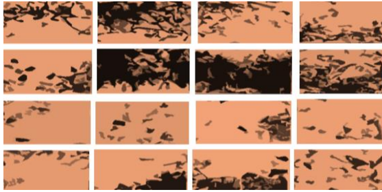
Şəkil 12. Konusvari matrisada sona yetməyən presləmə prosesindən sonra oxboyunca dördə-bir enkəsiyinin mikrostruktur, X400
