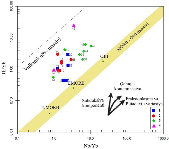
Şək. 5. Qabbro-tonalit formasiya süxurlarının fiqurativ nöqtələrinin Th/Yb-Nb/Yb diaqramında vəziyyəti 17 . İxtisar: NMORB - normal orta okean silsilə bazaltları; EMORB - zənginləşmiş orta okean silsilə bazaltları; OIB - okean adalarının bazaltları. Şərti işarələr: şəkil 4-də olduğu kimi
