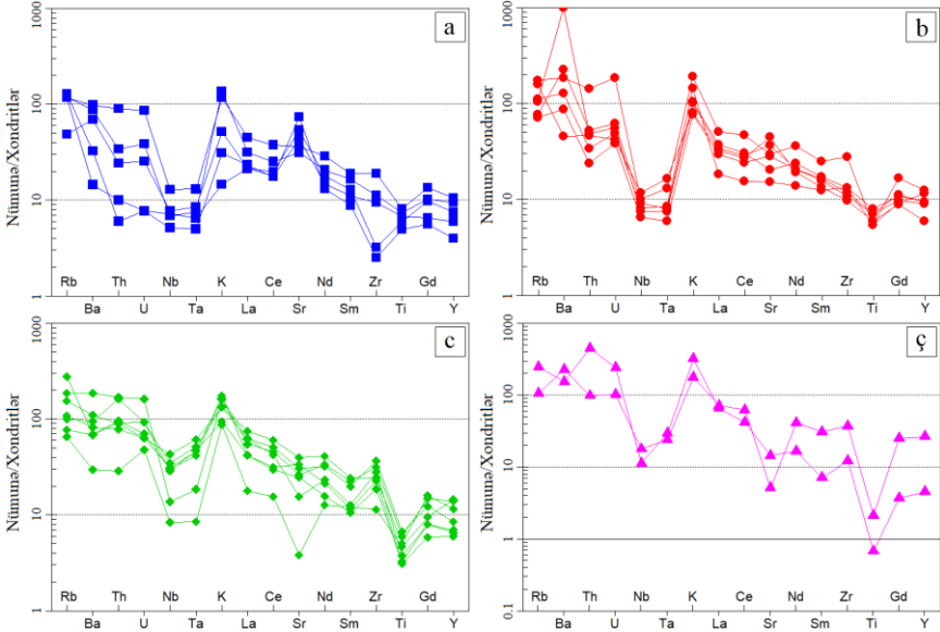
Şək. 2. Xondritə görə normallaşdırma diaqramları 9 : a) qabbroidlər; b) diorit-monsodiorit-kvarşlı dioritlər; c) tonalit-qranodioritlər; ç) qranit-aplitlər
