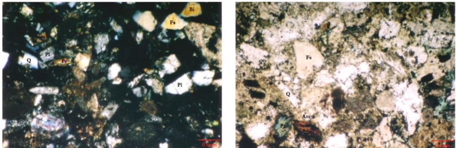
Q-kvars, Fs-çöl çpətı, Bi-biotit, Pl-plagioklas, Pr-Piroksen, Am-Amfibol
