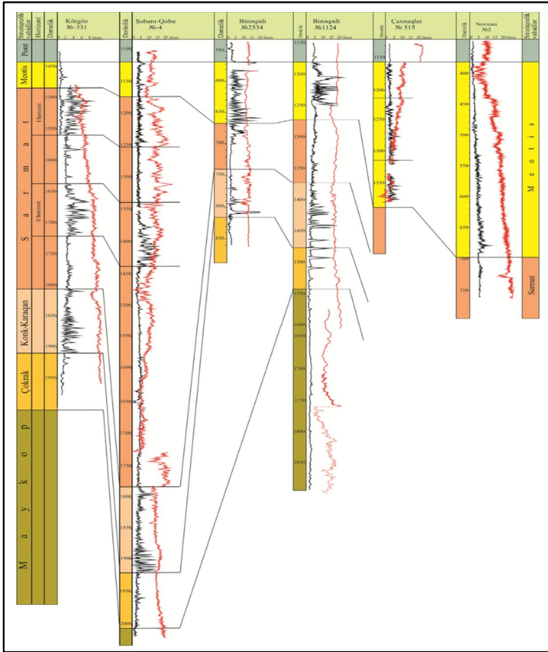
Şəkil 2. Fərqli sahələr üzrə Qərbi Abşeronun Miosen çöküntülərinin litostratigrafik xüsusiyyətlərinin müqayisə sxemi.
