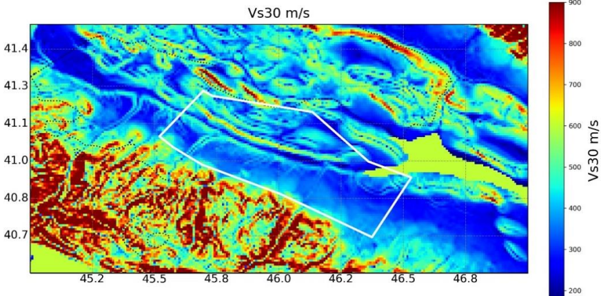
Şəkil 2. Tədqiqat ərazisinin V_{S30} xəritəsi (BŞTB 2 məlumatlarını emal edərək xəritəni tərtib etdi: T.H.Babayev)
