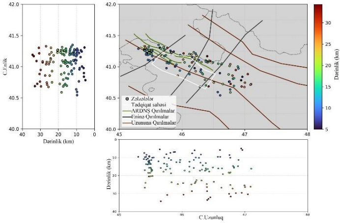
Şəkil 5. Zəlzələlərin qırılmalar üzrə episentral paylanması və dərinlik dəyişmələri (Tərtib etdi: T.H.Babayev)
