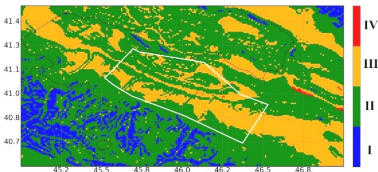
Şəkil 10. Tədqiqat ərazisinin qrunut təsnifatı xəritəsi. I, II, III və IV qrunut sinifləri xəritədə müvafiq rənglərlə göstərilmişdir (Tərtib etdi: T.H.Babayev)
