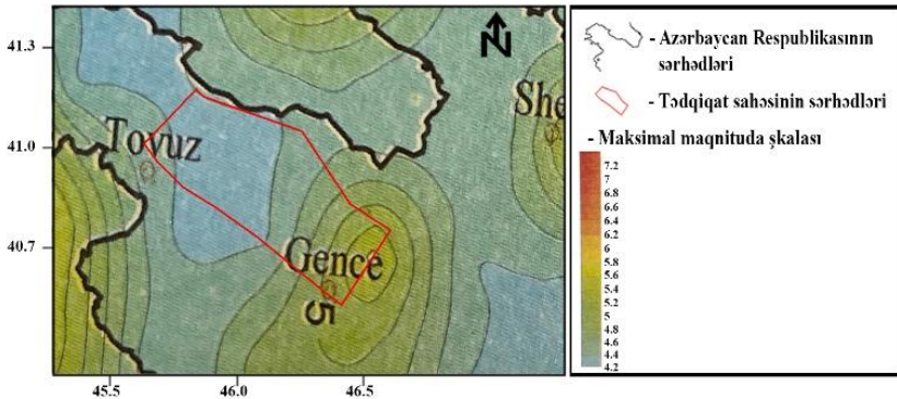
Şəkil 4. 1902-2010-cu illər kataloqu əsasında hesablanmış ehtimal edilən maksimal maqnituda xəritəsi (tərtib etdilər: F.Ə.Qədirov, Q.C.Yetirmişli, A.H.Qədirov 6 , işləyib və tədqiqat ərazisinə uyğunlaşdırıb: T.H.Babəyev)
