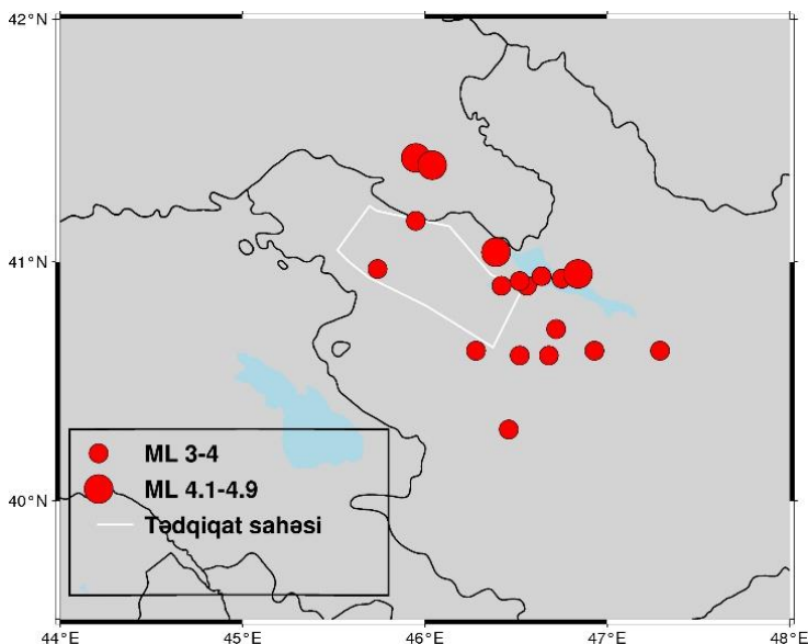
Şəkil 8. Zəlzələlərin maqnituda paylanması (Tərtib etdi: T.H.Babayev)
