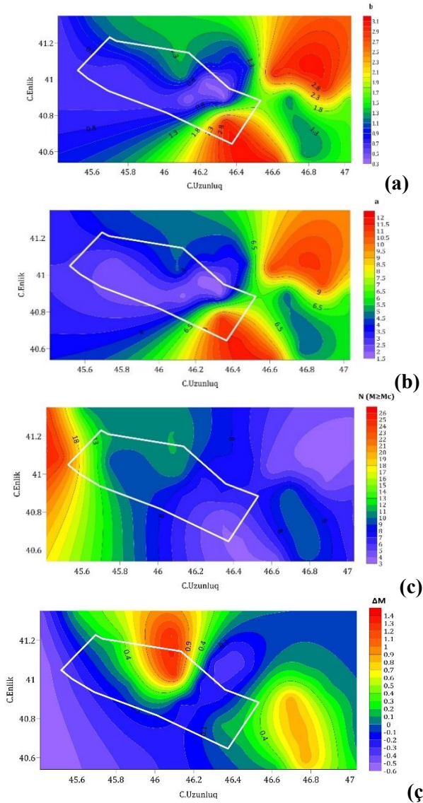
Şəkil 7. Kataloq üzrə hesablanmış seysmiklik indikatorlarının tədqiqat ərazisi üzrə paylanma xəritələri. (a) b ədədi. (b) a ədədi. (c) N: maqnitudası lokal maqnituda həddinin yekunlanma parametrinin təyin olunmuş qiymətindən böyük və ya bərabər olan zəlzələlərin sayı. (d) Maksimal maqnituda fərqi (Tərtib etdi: T.H.Babayev)
