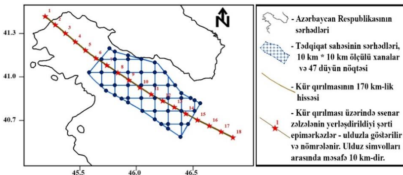
Şəkil 9. Ssenar zəlzələ üçün müəyyən olunmuş şərti episentrərlərin təsviri və tədqiqat sahəsinin seqmentləşdirilməsi (Tərtib etdi: T.H.Babayev)
