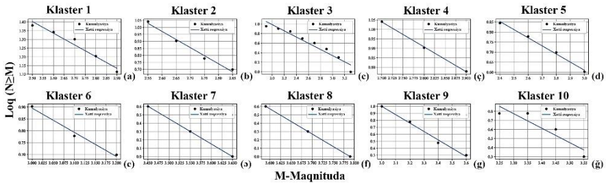
Qrafik 1. Klasterlər üzrə Q-R qanununun təsviri və b ədədinin xətti regressiya ilə hesablanması (Tərtib etdi: T.H.Babayev)
