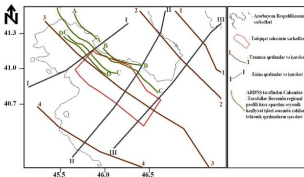
Şəkil 3. Tədqiqat ərazisi üzrə G.J.Yetirmishli et al. 3 , T.Babayev et al. [9] işlərinə və ARDNŞ-in 2011-ci il layihəsinin nəticələrinə 4 əsasən dissertasiya müəllifi tərəfindən tamamlanmış ümumiləşdirilmiş tektonik dərinlik qırılmaları xəritəsi (Verilənlər əsasında tərtib etdi: T.H.Babayev)
