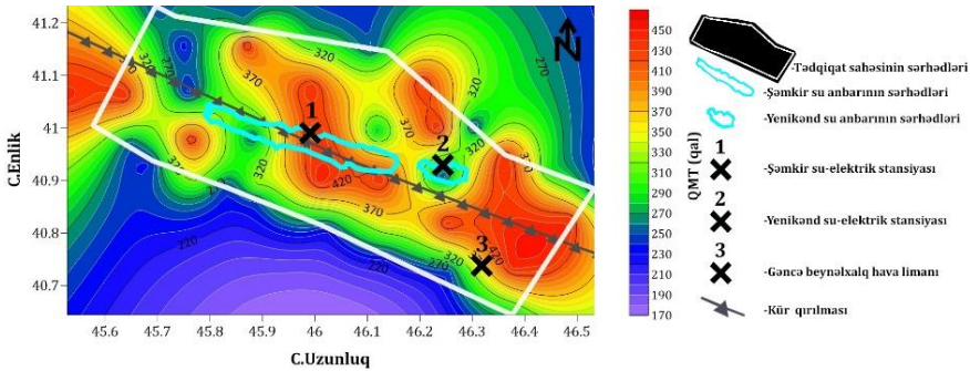
Şəkil 11. Tədqiqat sahəsi üçün müəyyən edilmiş “ən pis ssenari” ( M=6 ) üzrə proqnozlaşdırılan QMT paylanma xəritəsi (Tərtib etdi: T.H.Babayev)
