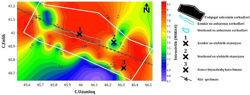
Şəkil 12. Tədqiqat sahəsi üçün müəyyən edilmiş “ən pis ssenari” (M=6) üzrə proqnozlaşdırılan QMT qiymətləri əsasında tərtib olunmuş intensivlik vahidlərində seysmik təhlükə xəritəsi (Tərtib etdi: T.H.Babayev)
