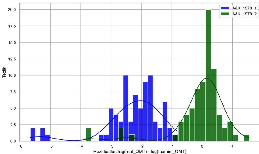
Qrafik 3. Reziduallar. Göy rəng A&K-1979-1 tənliyi, yaşıl rəng A&K-1979-2 tənliyi üçün (Tərtib etdi: T.H.Babayev)
