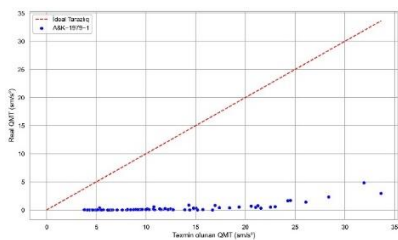
Qrafik 2. A&K-1979 tənlirlərinin proqnozlaşdırdığı QMT-nin tədqiqat sahəsi və yaxınlığında baş vermiş zəlzələlərin seysmik yazılarından alınan təcillə müqayisəsi. (a) A&K-1979-1. (b) A&K-1979-2 (Tərtib etdi: T.H.Babayev)
