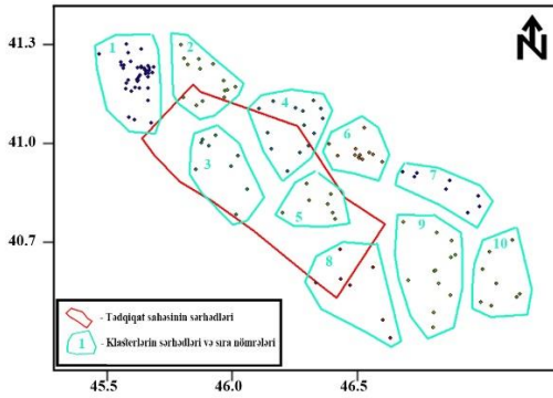
Şəkil 6. Kataloqun klasterlər üzrə episentral paylanması (Tərtib etdi: T.H.Babayev)
