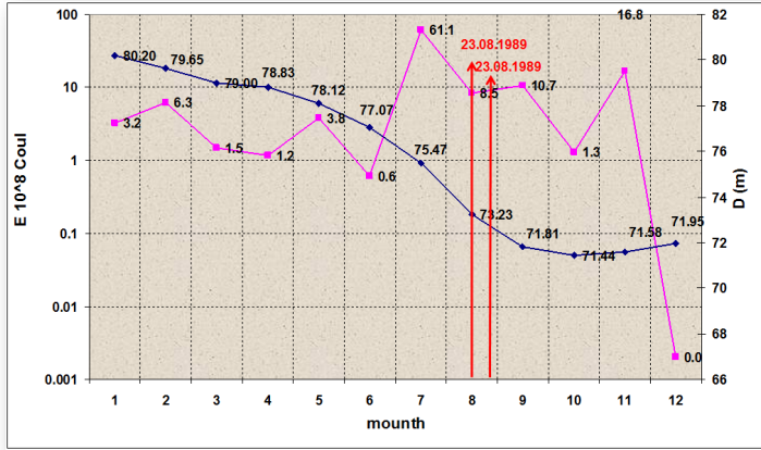
Şəkil. 10. 1989-cu il ərzində Mingəçevir su hövzəsində suyun dəyişməsi ilə baş vermiş zəlzələlər zamanı ayrılan enerjinin təsiri nəticəsində sürüşmə proseslərinin aktivləşməsi qrafiki
