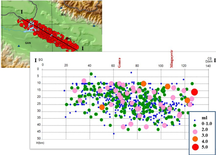
Şəkil. 5. Mingəçevir su hövzəsi ərazisinin I-I profili üzrə seysmoloji kəsilişi (2003-2017-ci illər)
