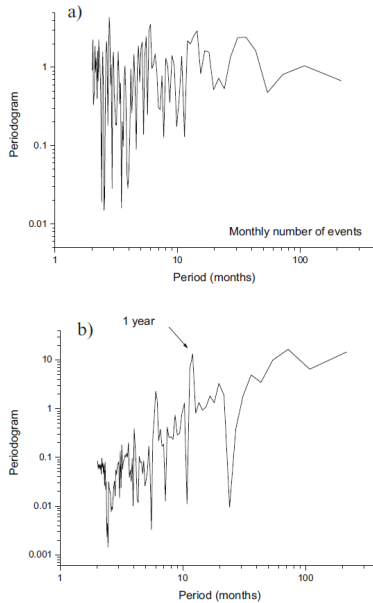
Şəkil. 8. Zəlzələ sayının (a) və suyun səviyyəsinin (b) aylıq periodogramının korreloqramması
